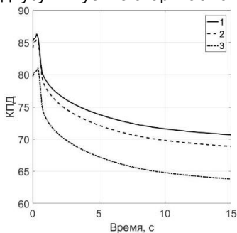
Рис. 2. Динамика КПД в процессе нагрева для одно- (1), двух- (2) и трех- (3) виткового индуктора
