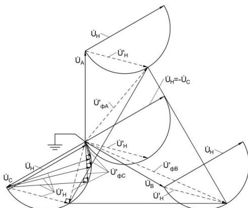
Рис. 2. Векторная диаграмма, построенная на основании результатов эксперимента на компьютерной модели
