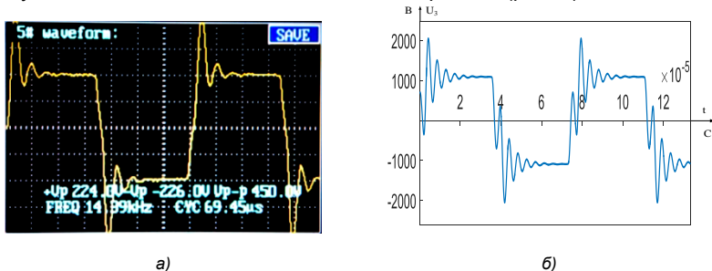
Рис. 3 Опытные (а) и расчетные (б) осциллограммы напряжения на кабельной линии при номинальной мощности нагрузки P_{\text{НОМ}1} = 1 кВт и P_{\text{НОМ}2} = 1,2 кВт: осциллографирование высокого напряжения производилось через делитель 1/10; осциллограммы в начальной, промежуточной и конечной точках линии практически не имеют отличий.
