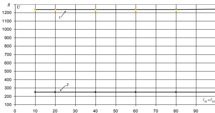
Рис. 2. Зависимости напряжения от длины участков l_{к1} и l_{к2} при P_{H1} = P_{H2} \cong 2 кВт: 1 – высокое напряжение в начале кабельной линии, в точке отбора и к конечной; 2 – напряжение на нагрузке в промежуточной и конечной точках
