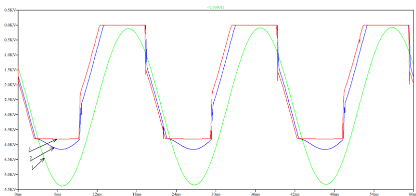
Рис.1. Изменение анодного напряжения при различных сопротивлениях системы «анод-катод»: 1 – температура катода 293К, сопротивление системы 8,113 \cdot 10^5 Ом; 2 – температура катода 1000К, сопротивление системы 76,615 Ом; 3 – температура катода 1593К, сопротивление системы «анод-катод» 13,3 Ом
