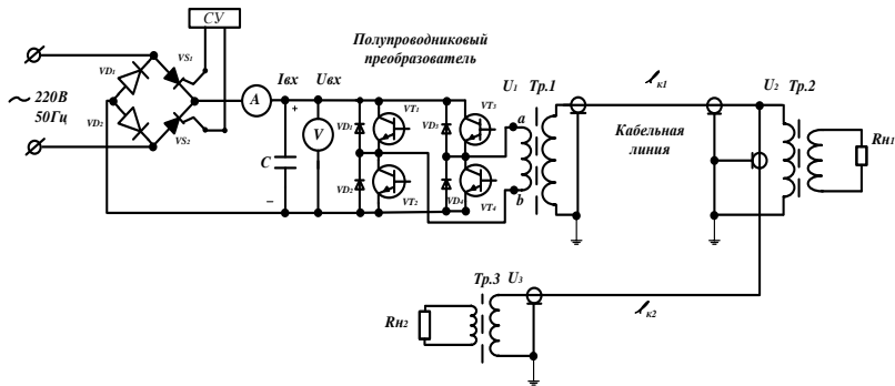
Рис. 1. Электрическая схема лабораторного макета ЭТКПЧ магистрального типа: где C – емкость на шинах постоянного тока для сглаживания пульсаций, VT1 - VT4 , VD1 - VD4 – силовые транзисторы и диоды (тиристоры) полупроводникового преобразователя соответственно, Tr1 , Tr2 и Tr3 – повышающий и два понижающих силовых трансформатора, l_{k1} и l_{k2} – длина участков кабельной линии, R_{H1} и R_{H2} сопротивление нагрузки в промежуточной и конечной точках
