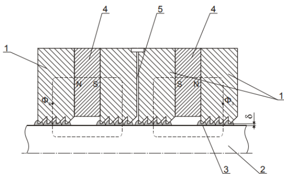
Рис.2. Конструкция магнитной цепи МЖГ. 1 – полюсные приставки; 2 – вал; 3 - магнитная наножидкость; 4 - Постоянные магниты; 5 - заправочный канал
